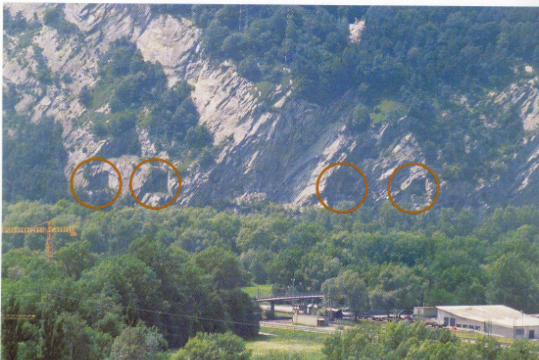
AW Haselboden: Blick des Mg 2 Richtung Trimmis (oben); Ansicht der 7,5 cm BK-Scharten (unten).
